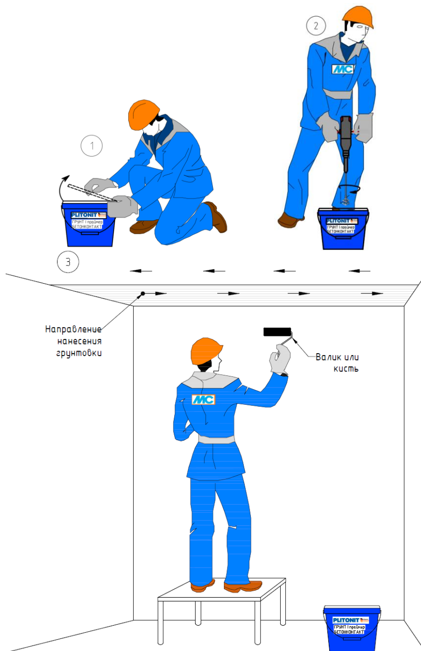
Рис.11. Последовательность работ.
