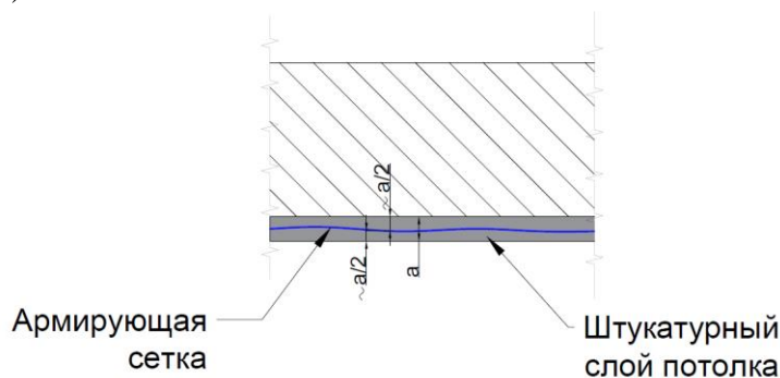
Рис. 15. Армированный штукатурный слой в местах стыка разных материалов и плит перекрытия
