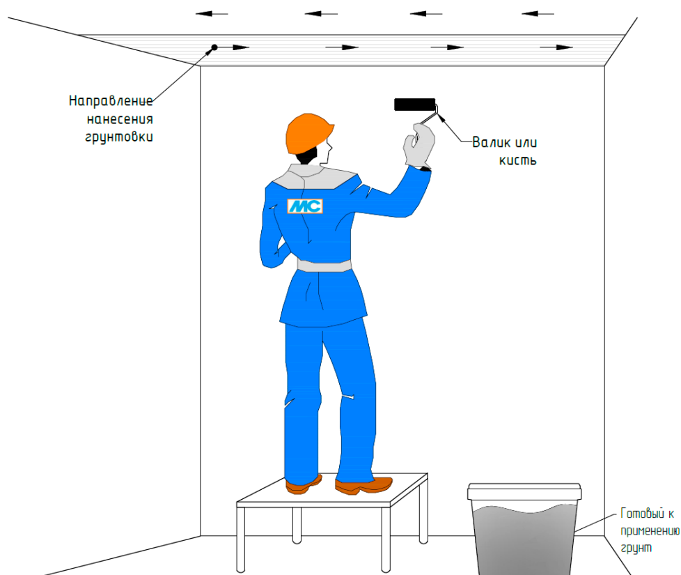
Рис. 16. Схема организации работ по нанесению грунта на основание
