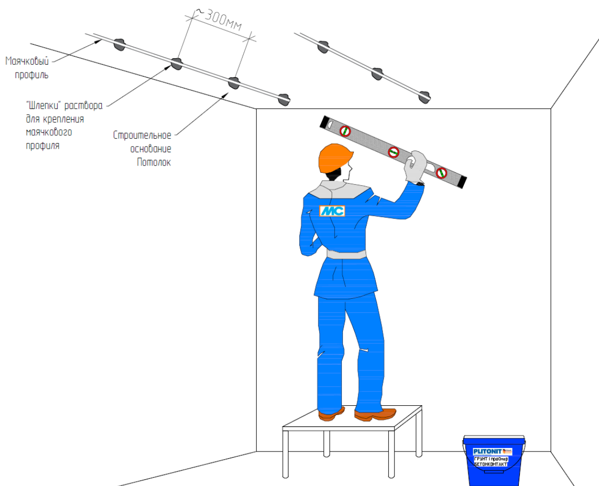
Рис.13. Монтаж маяка с помощью правила с уровнем
