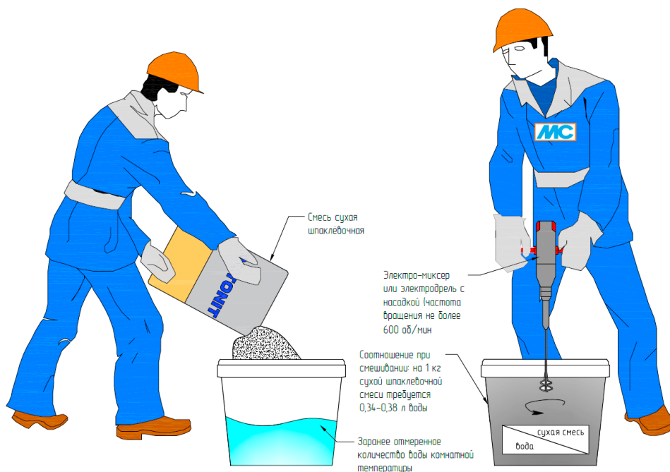
Рис. 17. Организация работ по затворению сухой шпаклевочной смеси
